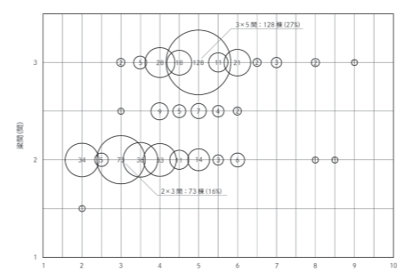
図2 平面規模
