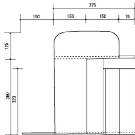
右側面図
