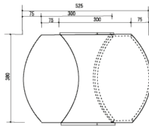
上面図
